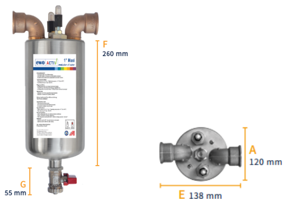
EWO® ACTIV 1" Maxi für 1.000 - 2.500 Liter Systeminhalt 2 STK. Magnesium Anoden
