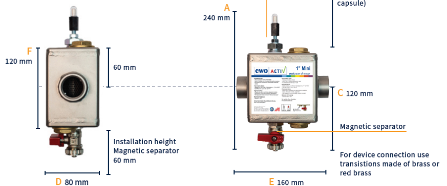
EWO® ACTIV 1" Mini for 100 - 400 liters system volume
